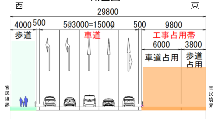
断面図
