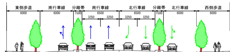
A-A断面図
